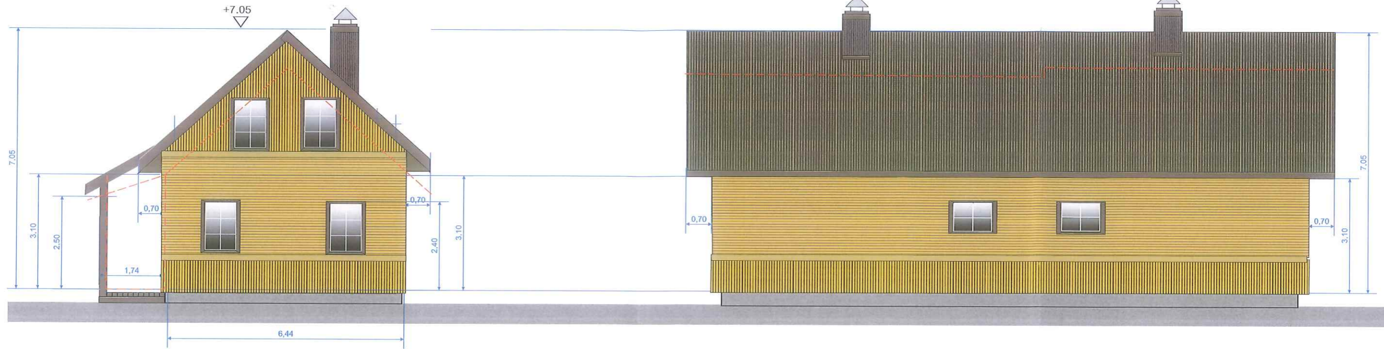
FASADAS TARP AŠIŲ 1-2
