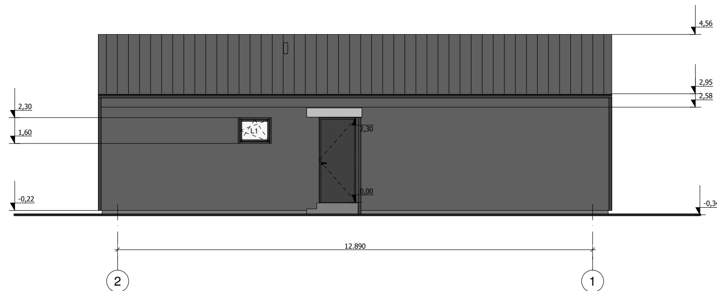
FASADAS 2-1, M 1:100
